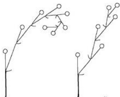
monochasial cymes
